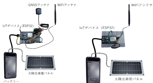
図4 検討した第4種踏切支援装置 (左：車上装置、右：地上装置)
