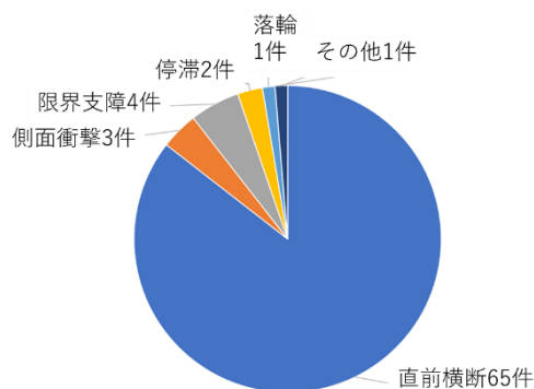
図3 第4種踏切の自動車等における事故原因（3年間）
