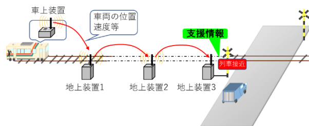
図5 第4種踏切支援装置の動作イメージ
